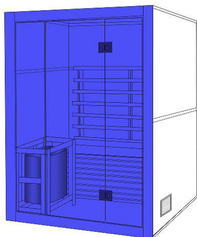
(9) namestite sprednji panel in ga pritrdite z zunanjiimi sponkami
