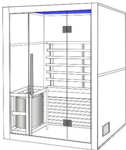
(11) postavite stropni panel na ostale dijelove kabine i spojite konektore na krovu
