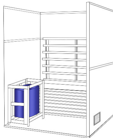
(8) peč vstavite v zaščito po navodilih za uporabo peči
