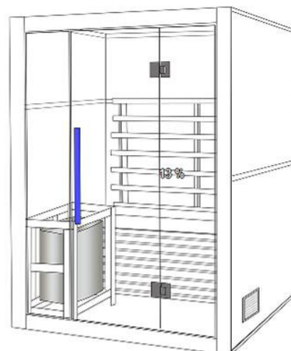
(10) namestite ročaj in tesnila
