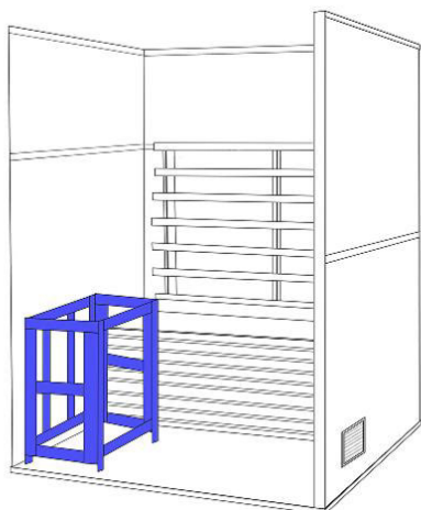
(7) pričvrstite zaštitu peći vijcima M3.5*40
