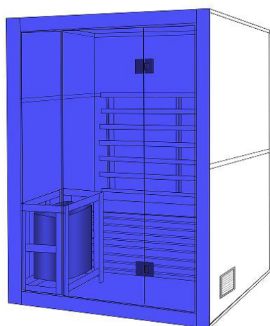
(9) postavite prednji panel na lijevi i desni panel i pričvrstite ga vanjskim kopčama
