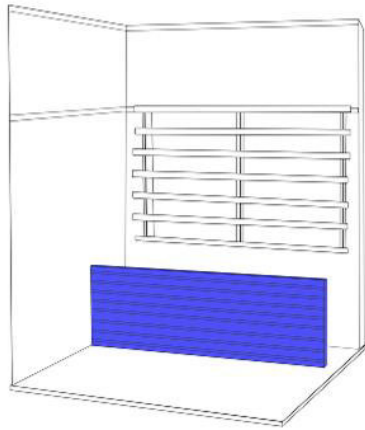
(5) podporor za klop postavite na talni panel Tako, da sede v reže med lesene letvice
