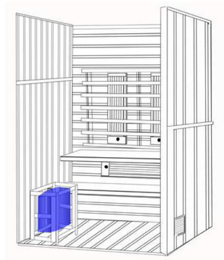
(8) Montieren Sie den Saunaofen auf das Gitter gemäß Handbuch für den Ofen.
