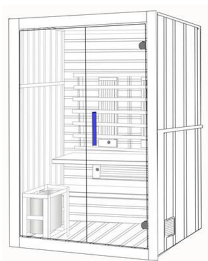
(11) postavite ručku i brtvu za staklo na vratima
