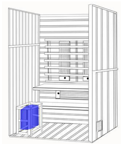
(8) peč za savno namestite v zaščito peči v skladu s priročnikom za peč
