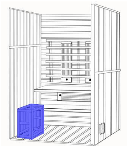
(7) sastavite zaštitu peći (vijcima M3,5*40)
