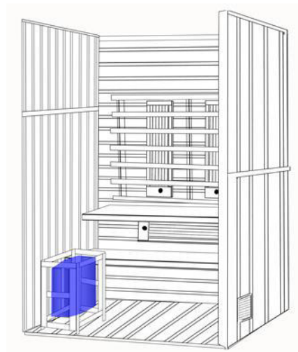
(8) stavite peć u zaštitu prema uputama za korištenje peći
